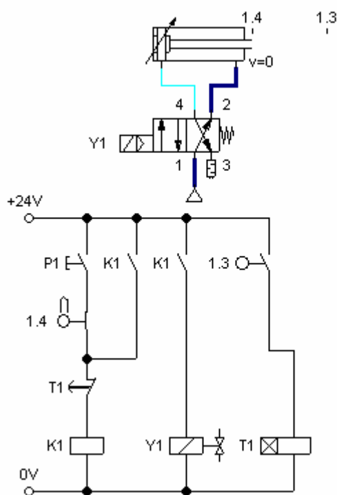
Rys. 1. Układ elektropneumatyki
