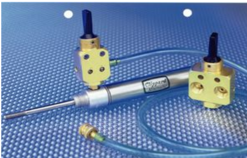
Rys. 2. Siłownik pneumatyczny z elementami przyłączeniowymi
