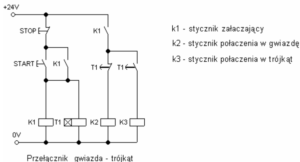
Rys. 11 przełącznik gwiazda - trójkąt
