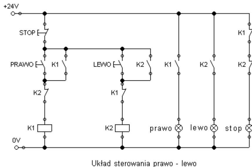
Rys. 10 Układ sterowania prawo - lewo
