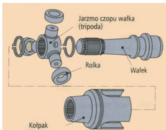
Rys. 31. Przegub tripodowy
