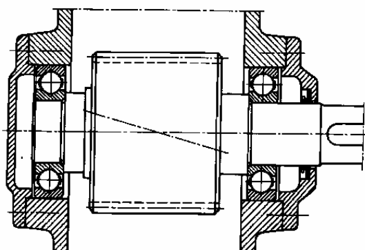
Rys. 19. Dwustronne ustalenie wału
