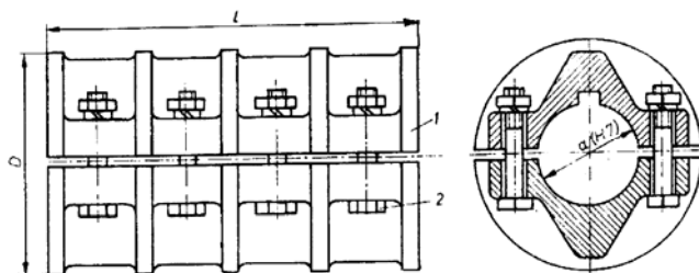
Rys 22. Sprzęgło sztywne łubkowe; 1- łubki, 2-śruby
