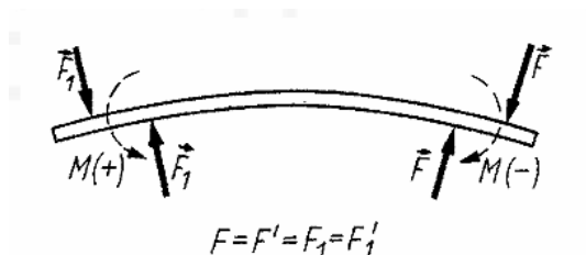
Rys. 3. Czyste zginanie
