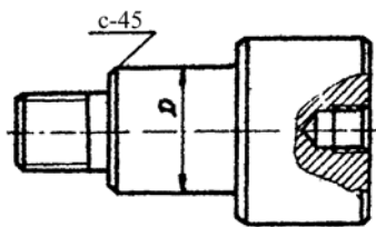
Rys. 12. Przykład fazki
