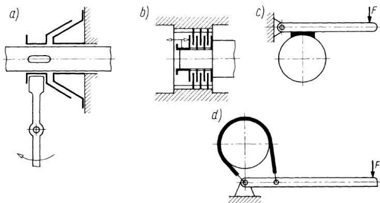
Rys. 34. Hamulce: a) stożkowy, b) wielopłytkowy, c) jednoklockowy, d) cięgnowy
