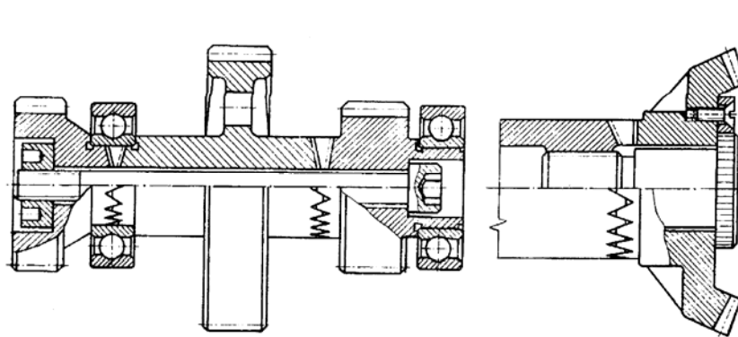
Rys. 27. Przykłady połączeń wieloząbkowych
