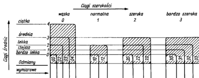
Rys. 15. Ciagi odmian średnic i szerokości łożysk
