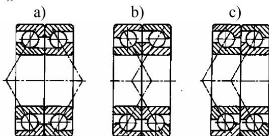
Rys. 16. Układy łożysk: a)-układ 0, b)-układ X, c)-układ tandem
