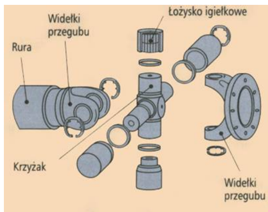
Rys. 30. Sprzęgło Cardana
